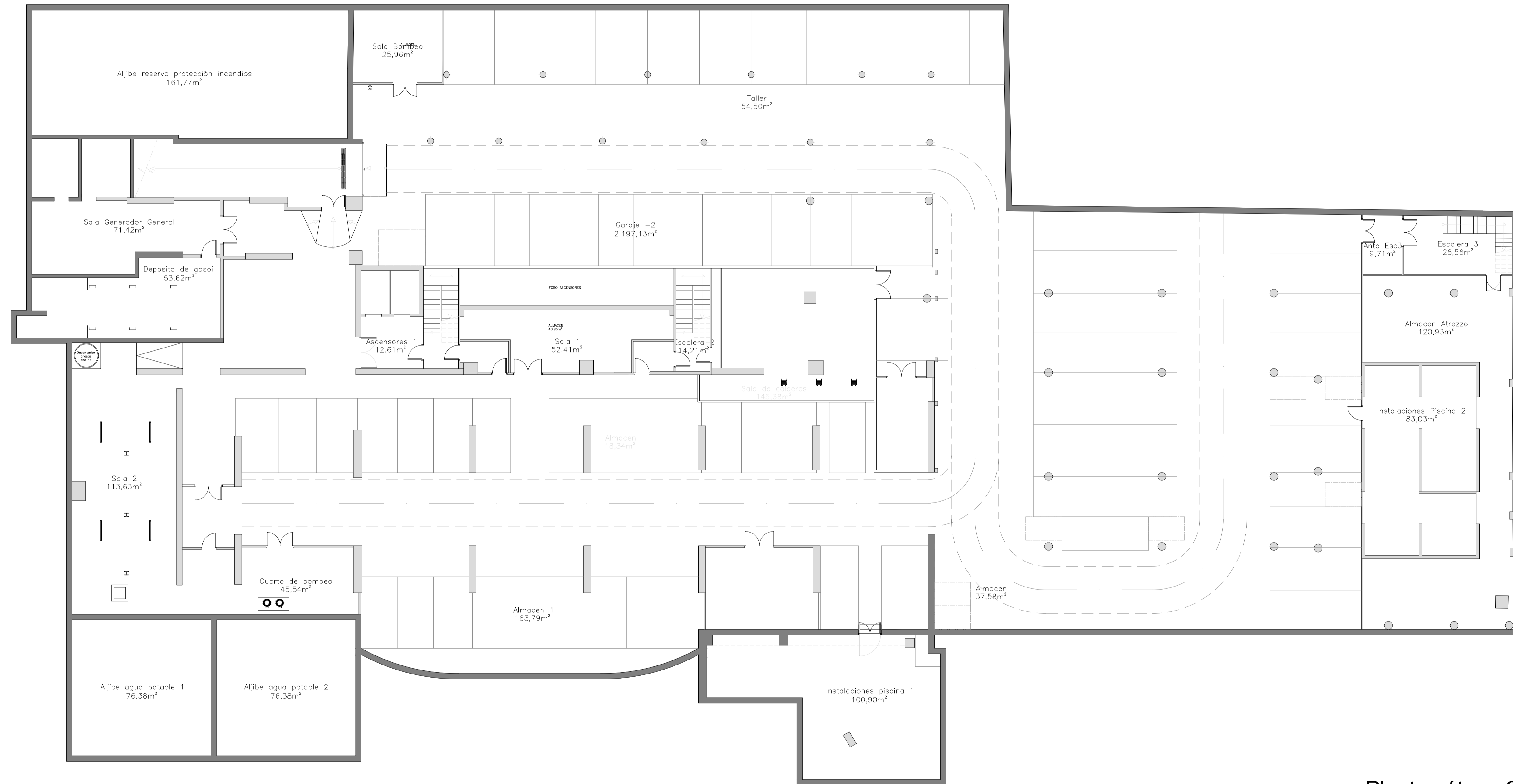
Planta sótano 2. Propuesta aparcamiento e: 1/150
